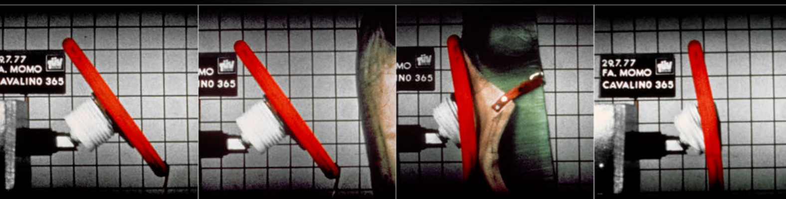
Impact test of the "dummy" against the assembly: wheel-hub-car, shows a perfect interaction of energy absorbtion forces. Prove d'urto del manichino contro il sistema "volante-mozzo-vettura", dimostrano un'efficiente interazione degli assorbimenti di energia.
